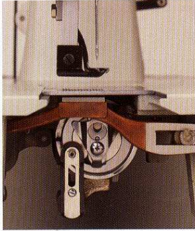
大旋梭、上下同步送料，使缝制厚料更轻松。
